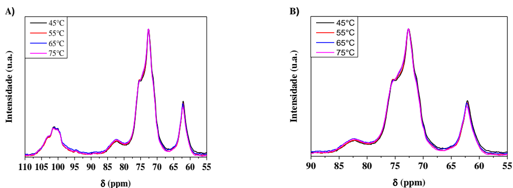
Figura 7: Sinais obtidos pelo método de CP-MAS de farinhas de batata-doce biofortificada secas a 45; 55; 65 e 75°C.
